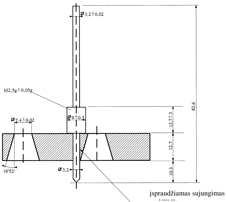
1 pav. Penetrometras
